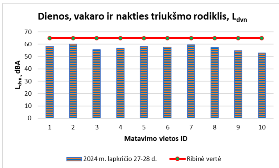
43 pav. Dienos, vakaro ir nakties triukšmo rodiklio ( L_{dvn} ) pasiskirstymas matavimo vietose.
