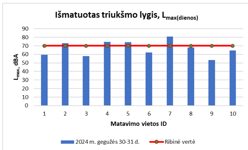
21 pav. Maksimalaus triukšmo lygio pasiskirstymas matavimo vietose dienos metu (7 – 19 val.).
